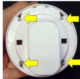
4 Schrauben rausdrehen
