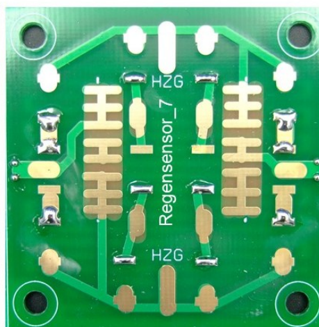
einseitig Lötunkte für die 12 SMD-Widerstände setzen
