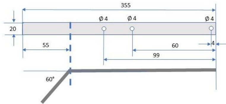
Bohrschema und Abkantung Alu-Flachmaterial 20x5
